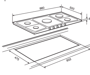
EX/90 5G AI AL TR EX/90 5G AI AL PC
