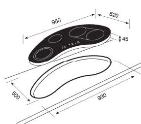
GKST-95 N I4 Select
