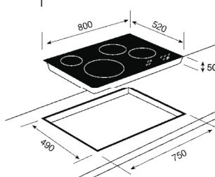
GKST-80 I4 Profi
