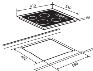
CG Lux 60 4G AI AL BUT CG Lux 60 4G AI AL NAT
