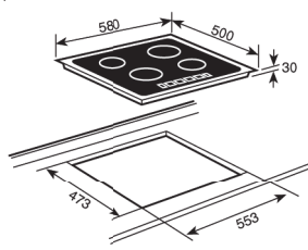
EF/60 2P 2G AI AL BUT EF/60 2P 2G AI AL NAT
